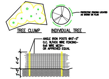
14 L5 Tree Protection Detail N.T.S.
