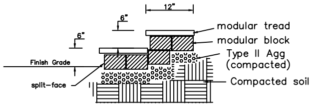
15 L5 Pathway Step Detail N.T.S.
