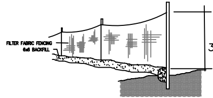
13 L5 Silt Fence Detail N.T.S.
